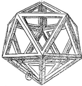
Octaèdre
