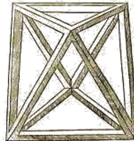
Tétraèdre
