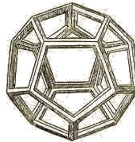
Dodécaèdre
