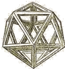
Isocaèdre
